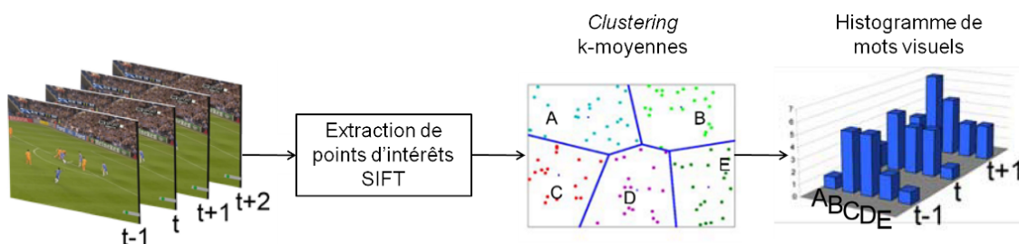
FIGURE 4.3 – Caractéristiques visuelles introduites par Ballan et al. [BBBS09] : Chaque vidéo est représentée par une séquence d’histogrammes de mots visuels. Illustration sur un exemple de la base MICC-Soccer-Actions-4 .
