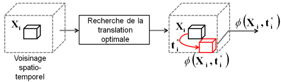
FIGURE 6.4 – Principe de la recherche de la translation optimale : Tous les patchs situés dans un certain voisinage spatio-temporel de X_i seront représentés par un seul patch translaté \phi(X_i, t_i^*) .
