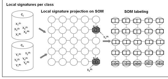
Figure 3. SOM labeling.
