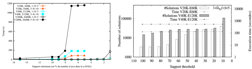
FIGURE 8: Performances des deux algorithmes pour les données artificielles (5 couches).
