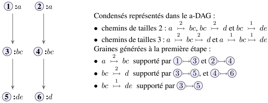
FIGURE 3: Exemple de motifs condensés non générés a \xrightarrow{1} bc \xrightarrow{1} de .
