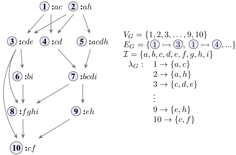
FIGURE 2: Exemple de a-DAG.
