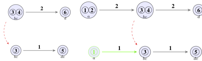
FIGURE 4: Exemple du backtracking pour générer a \xrightarrow{1} bc \xrightarrow{1} de .
