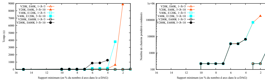
FIGURE 7: Performances et nombre de solutions en fonction des seuils de fréquence ( en %).
