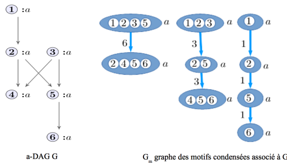
FIGURE 5: Graphe de motifs du a-DAG G : a \xrightarrow{6} a, a \xrightarrow{3} a \xrightarrow{3} a et \xrightarrow{1} a \xrightarrow{1} a \xrightarrow{1} a
