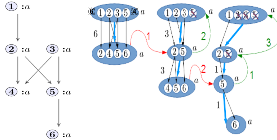
FIGURE 6: Etapes de construction du graphe de motifs du a-DAG à gauche
